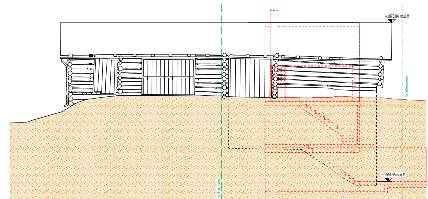
Nordfassade
