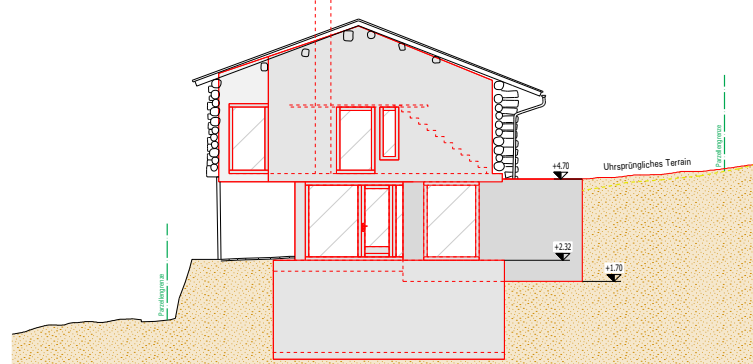
Ostfassade mitte Stallgebäude
