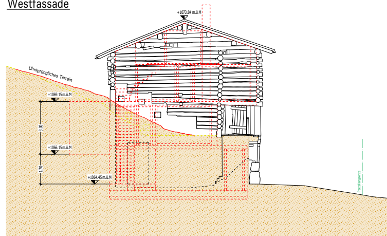
Westfassade
