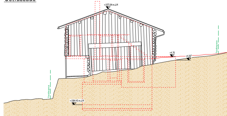
Ostfassade mitte Stallgebäude
