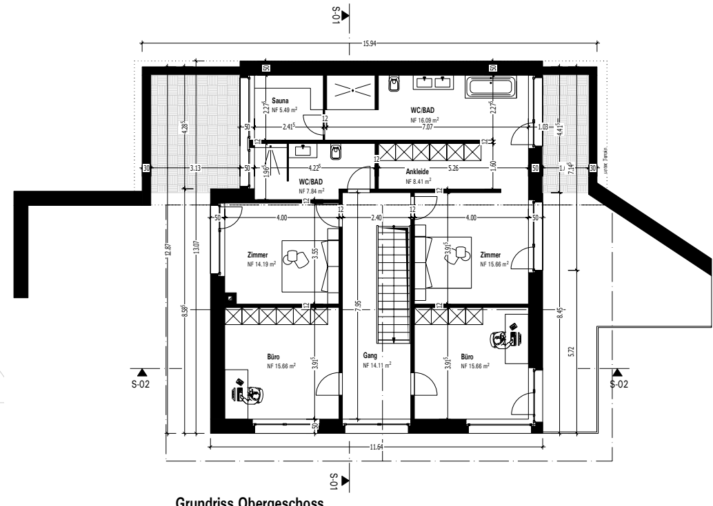
Grundriss Obergeschoss
