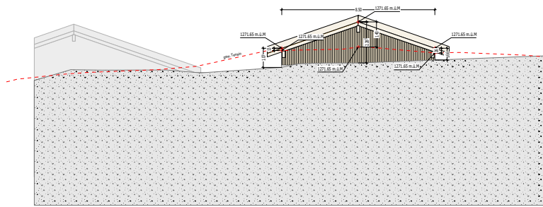
Nordfassade
