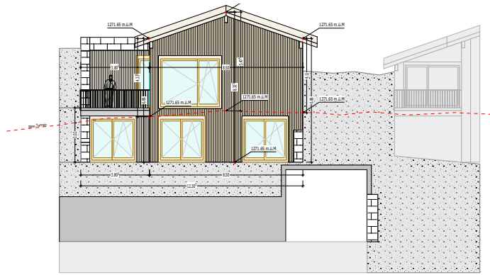
Südfassade
