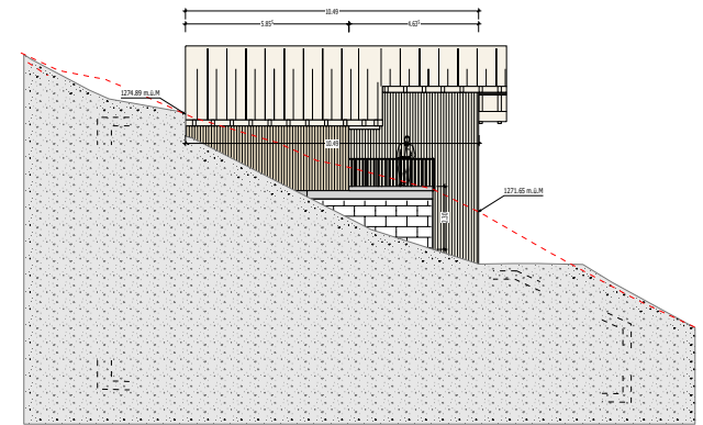
Westfassade
