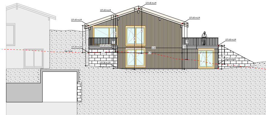
Südfassade
