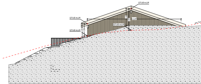
Nordfassade
