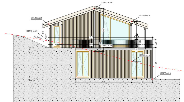
Westfassade
