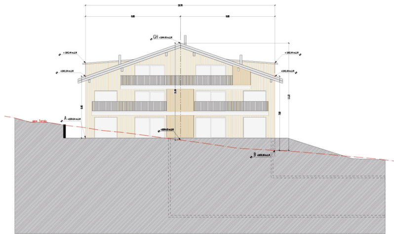
Südfassade
