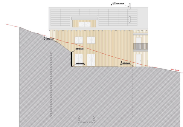
Westfassade
