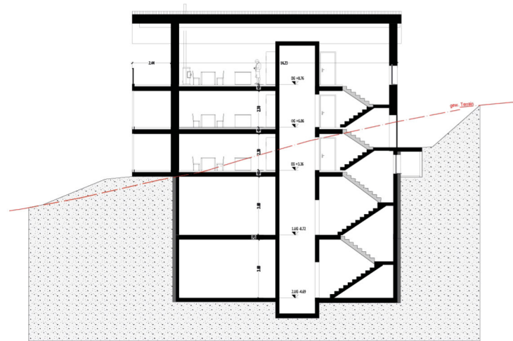
Schnitt S-03 Gebäude B
