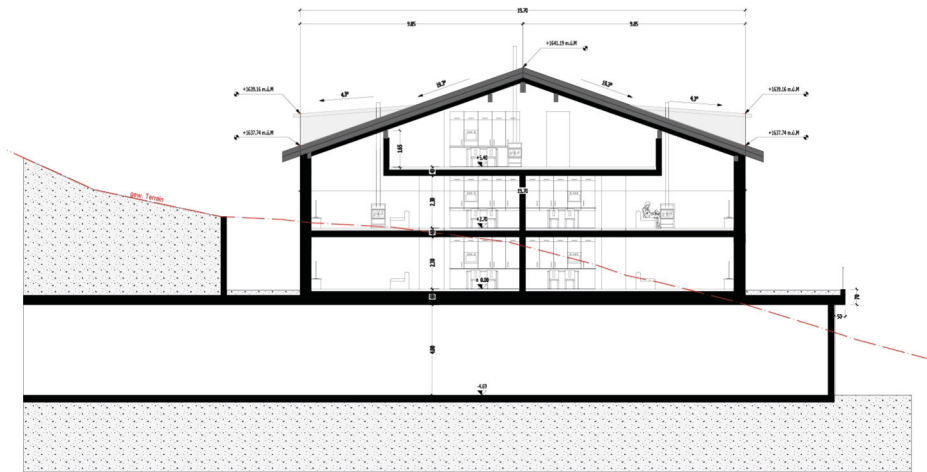
Schnitt S-02 Gebäude A
