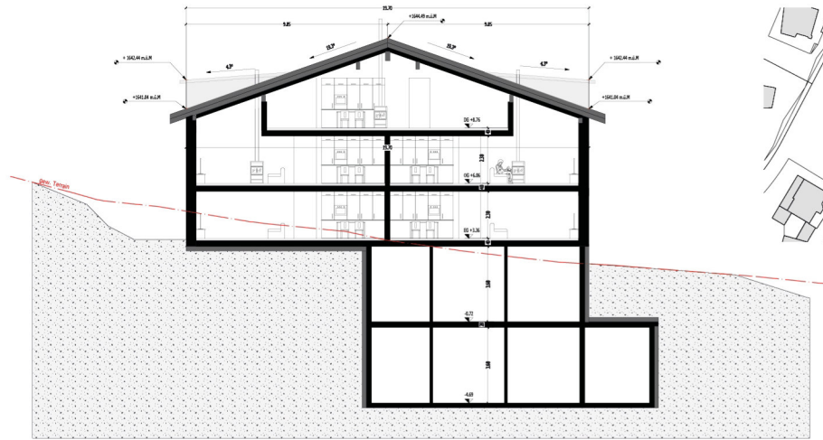
Schnitt S-04 Gebäude B
