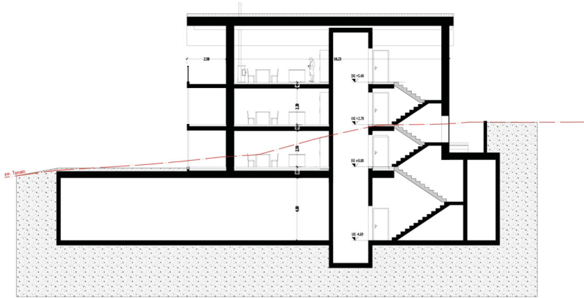
Schnitt S-01 Gebäude A
