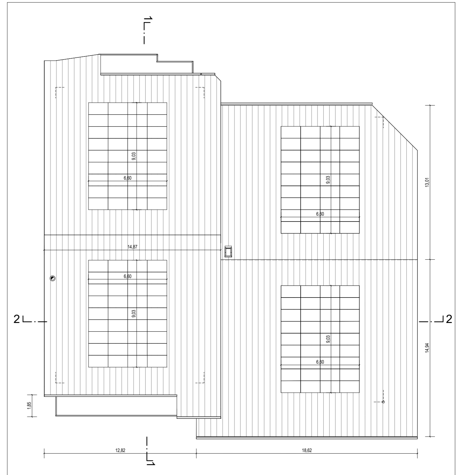
Dachansicht Photovoltaikmodule
